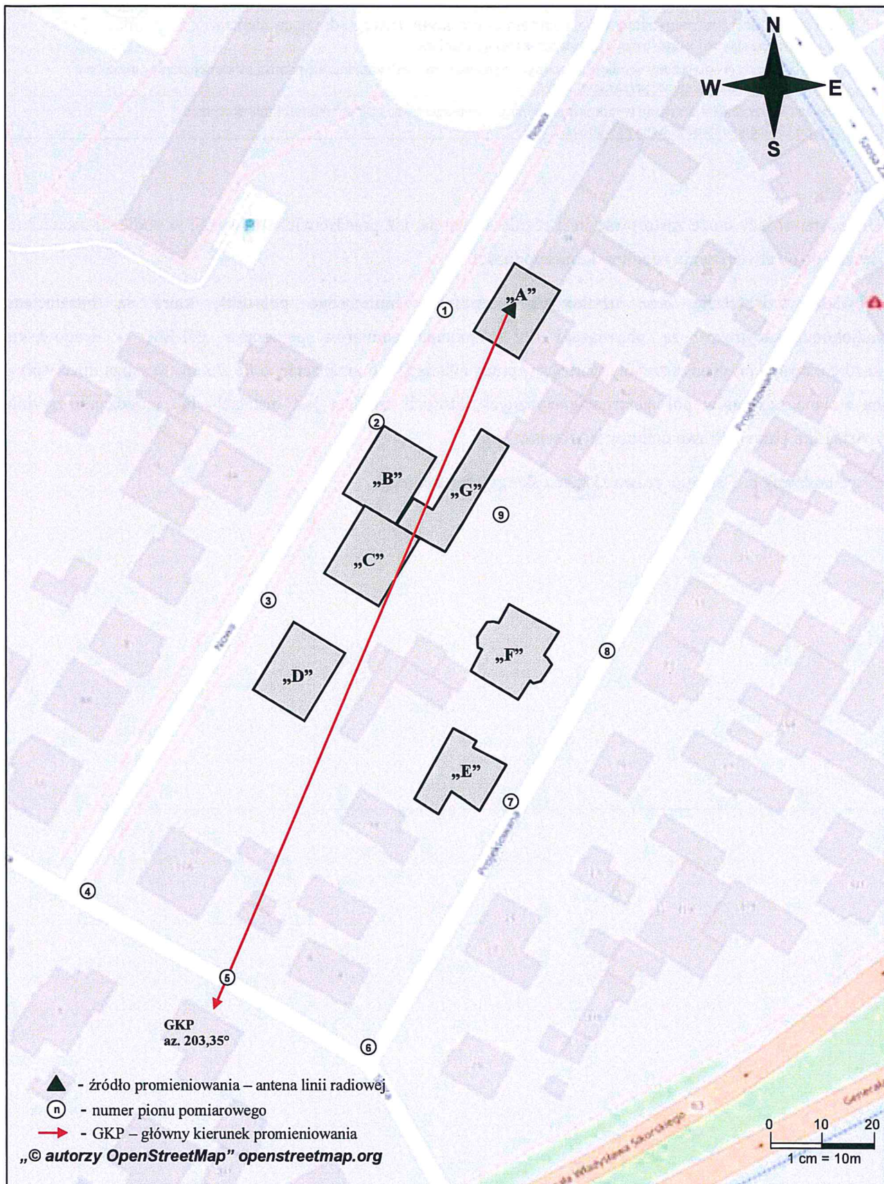
Rys. 1. Usytuowanie punktów i pionów pomiarowych w otoczeniu instalacji radiokomunikacyjnej Stacja Netia LOMZB055-LOMZM00058 Łomża, ul. Nowa 3A
