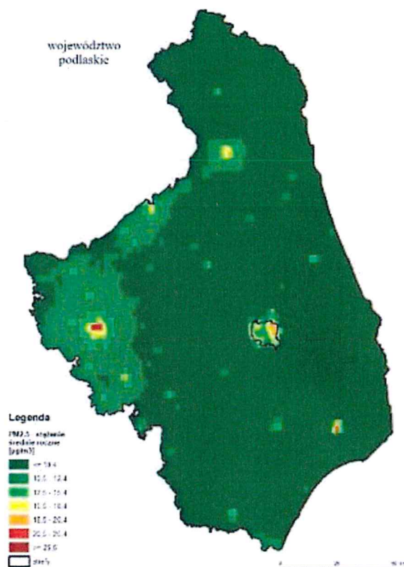
Rysunek 11. Rozkład przestrzenny wartości stężenia średniego rocznego pyłu PM_{2,5} w województwie podlaskim w 2020 r., opracowany z wykorzystaniem metody obiektywnego szacowania w oparciu o wyniki modelowania.
