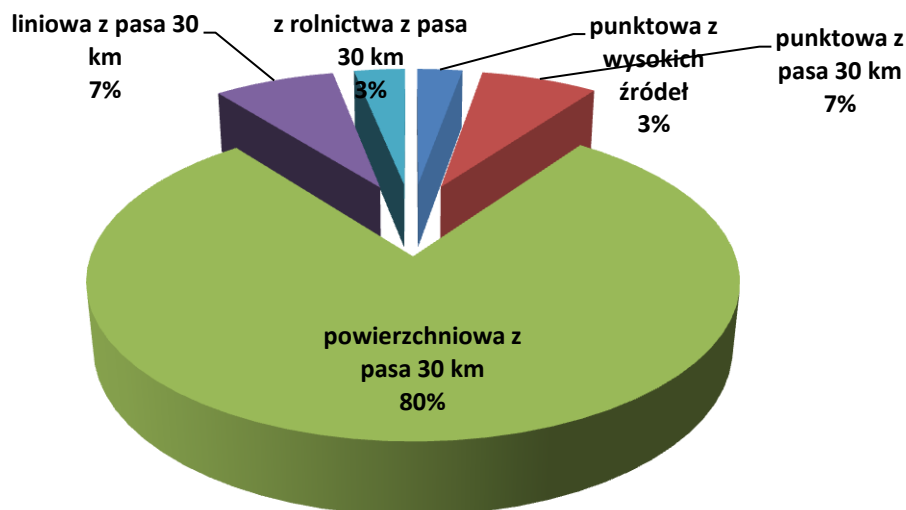
Rysunek 73 Udział procentowy emisji pyłu zawieszzonego PM 2,5 poszczególnych typów poza strefą podlaską w 2012 r.
