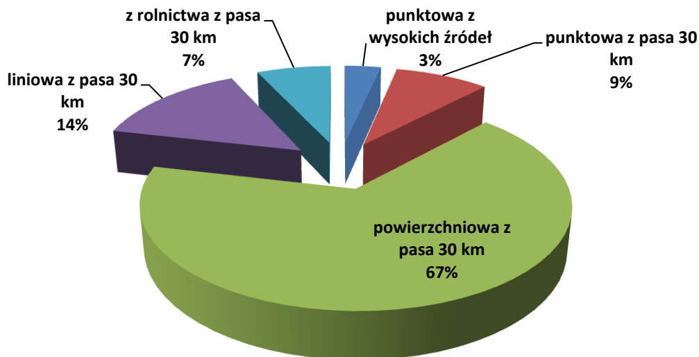
Rysunek 32 Udział procentowy emisji pyłu zawieszonego PM10 poszczególnych typów poza strefą podlaską w 2012 r.
