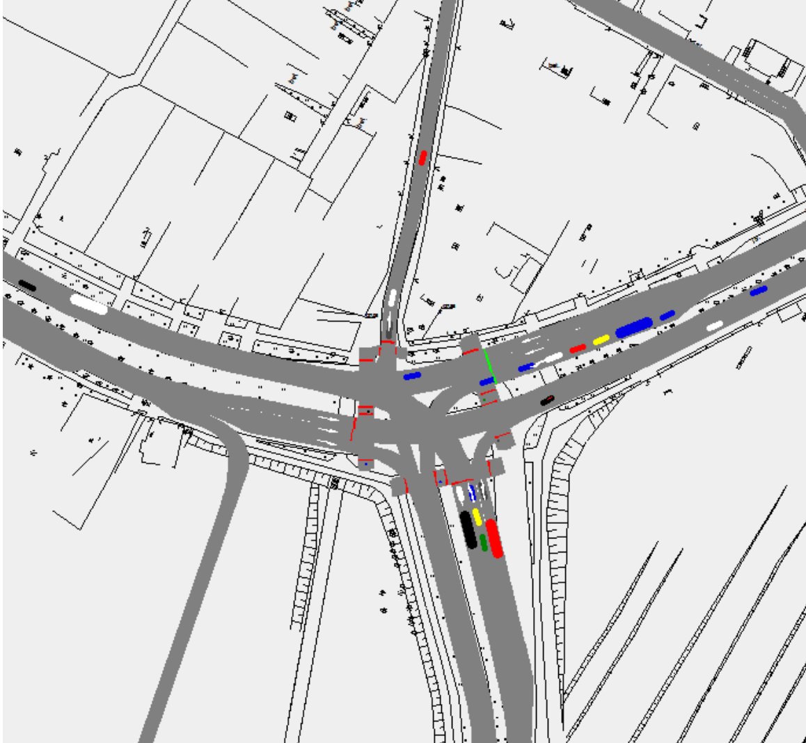
Rys. 28. Obraz ruchu na skrzyżowaniu ul. Sikorskiego i Zawadzkiej – długości kolejki pojazdów na skrócie w lewo w ul. Zawadzka w chwili włączenia sygnału zielonego dla tej relacji
