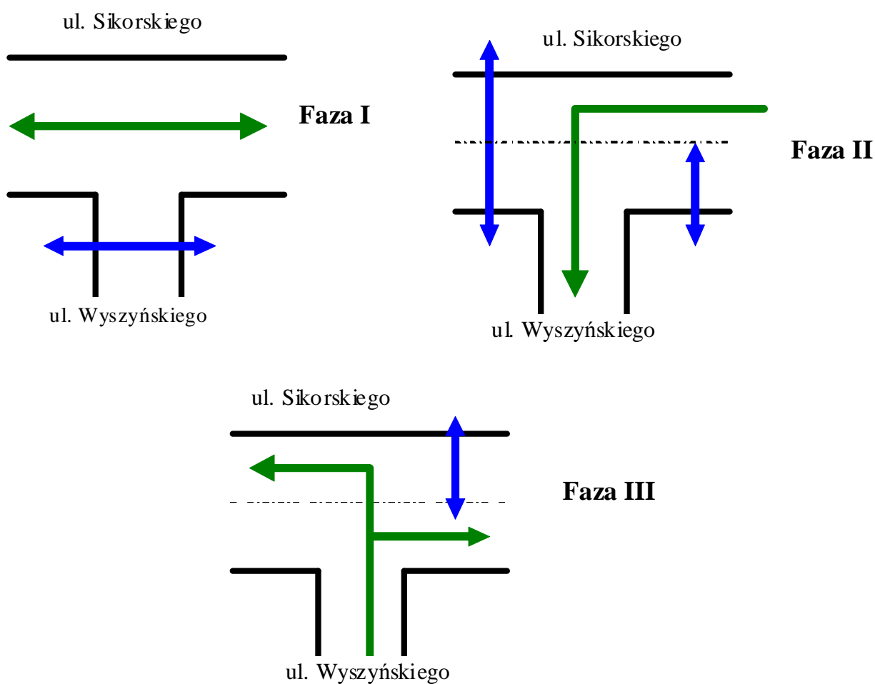
Rys. 24. Skrzyżowanie ul. Sikorskiego i Wszyńskiego – układ faz sygnalizacji świetlnej.
