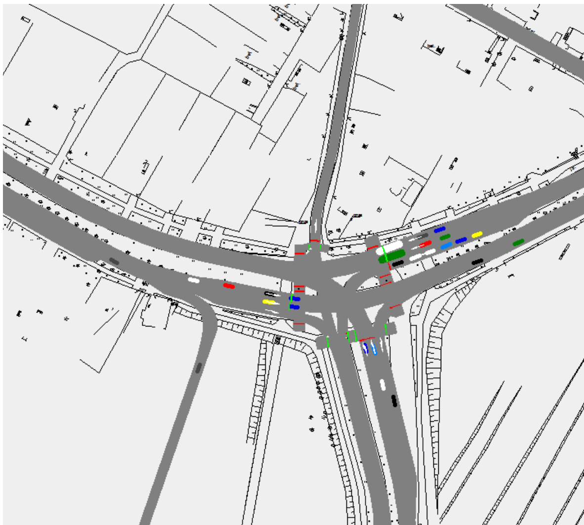
Rys. 31 Obraz ruchu na skrzyżowaniu ul. Sikorskiego i Zawadzkiej – liczba pojazdów oczekujących na jazdę na wprost wzdłuż ul. Sikorskiego w chwili włączenia sygnalu zielonego dla tego kierunku ruchu.
