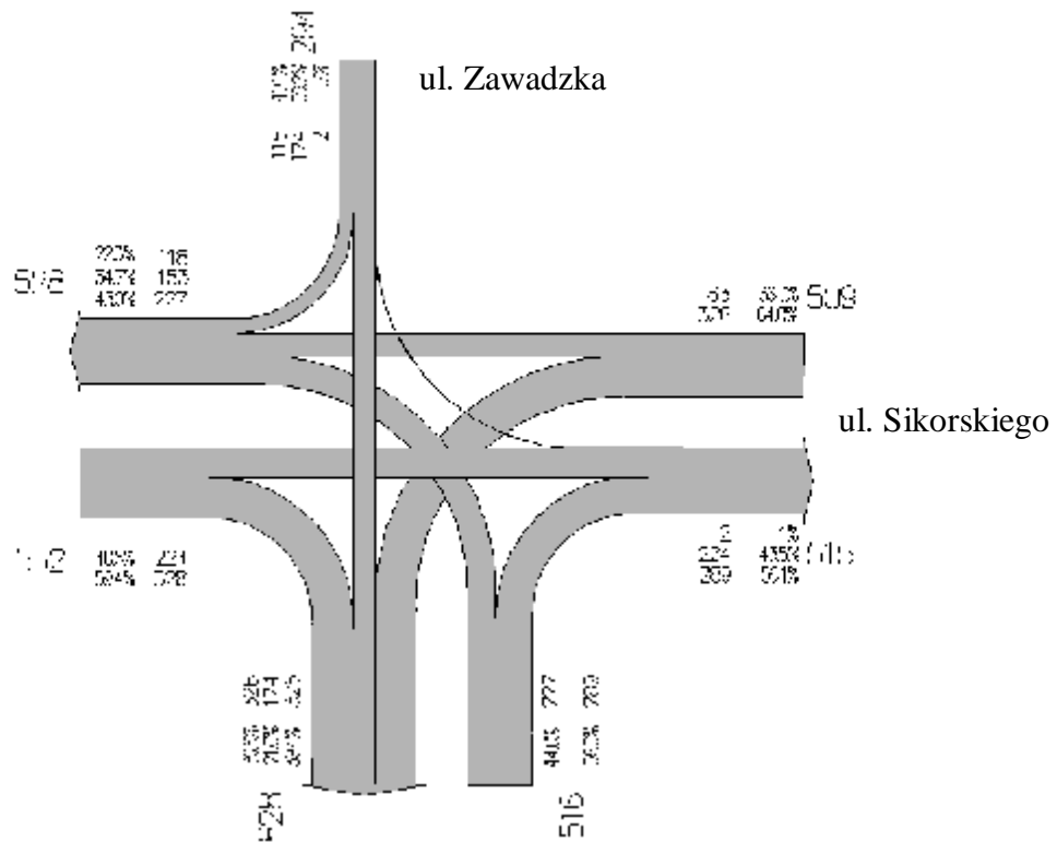
Rys. 9 Kartogram natężenia ruchu na skrzyżowaniu ul. Zawadzkiej i Gen. Sikorskiego – samochody osobowe (szczyt popołudniowy - godzina 15.00-16.00).
