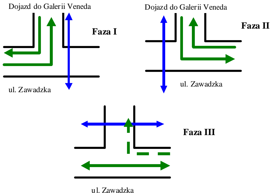
Rys. 20. Skrzyżowanie ul. Zawadzkiej i drogi dojazdowej do Galerii „Veneda” – układ faz sygnalizacji świetlnej.
