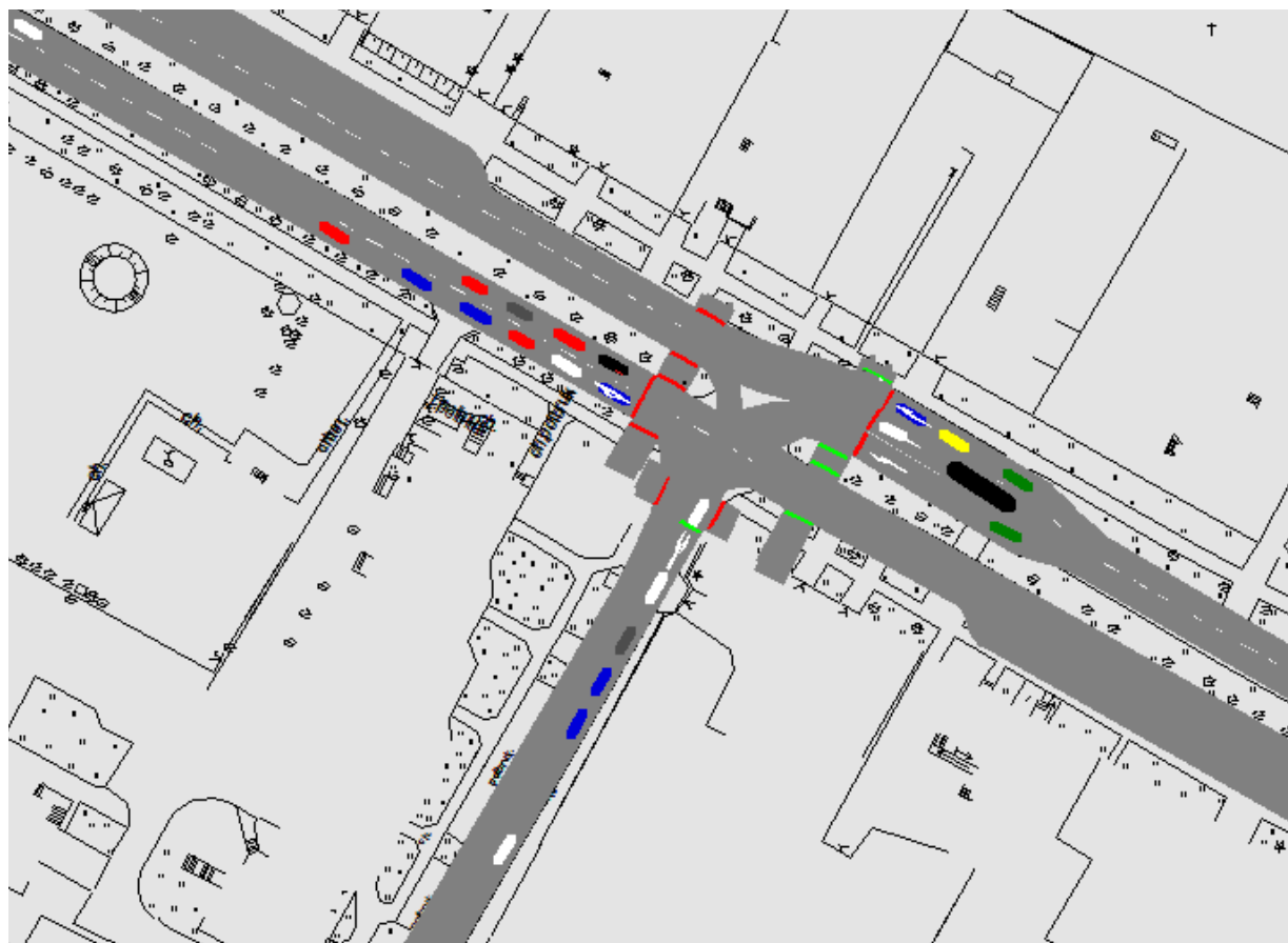
Rys. 33. Obraz ruchu na skrzyżowaniu ul. Sikorskiego z ul. Wyszyńskiego – liczba pojazdów oczekujących na wlocie ul. Kard. S. Wyszyńskiego w chwili włączenia sygnału zielonego dla tej relacji.
