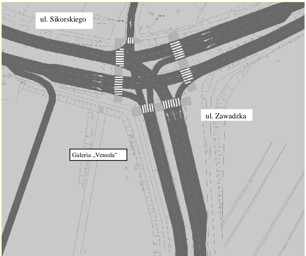
Rys. 21 Schemat organizacji ruchu na skrzyżowaniu ul. Zawadzkiej z ul. Sikorskiego.
